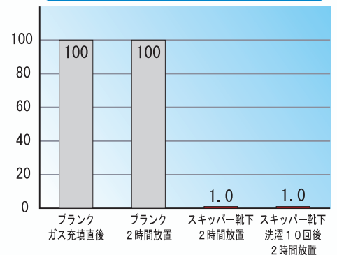
イソ吉草酸ガスの除去性能評価(減少率:%)
