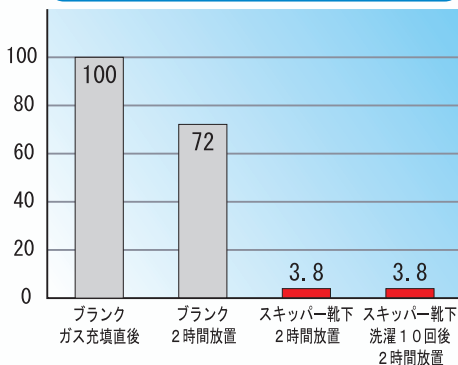
アンモニアガスの除去性能評価(残留濃度:ppm)
