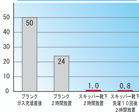
酢酸ガスの除去性能評価(残留濃度:ppm)
